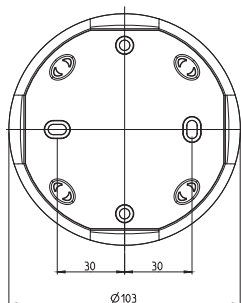
thePrema S360 KNX UP con telaio a vista 110A
